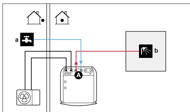
A Nádrž teplej vody pre domácnosť a PRÍVOD studenej vody b ODVOD teplej vody
