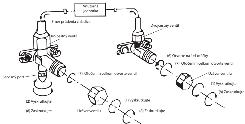
Schéma trojcestného ventilu
