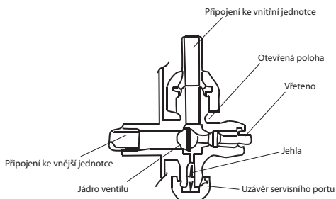
Schéma třícestného ventilu
