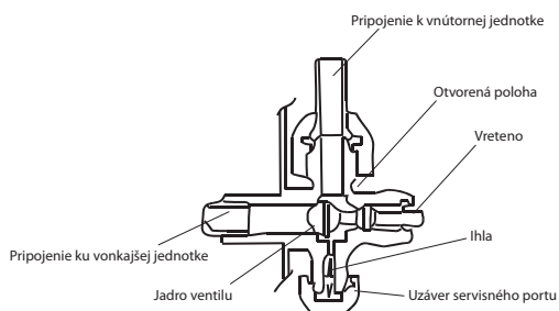
Schéma trojcestného ventilu
