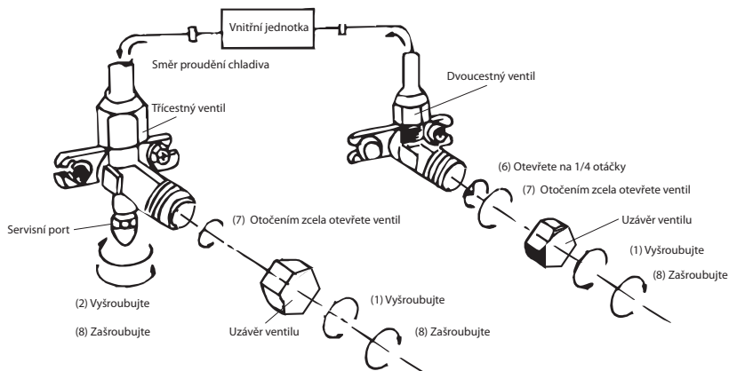
Schéma třícestného ventilu
